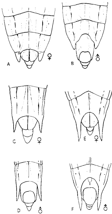
Fig. 1. Segmentos abdominales inferiores de Gerris sp., mostrando las puntas espinosas laterales del 7° segmento, y los segmentos genitales. A y B. G. costai . C y D. G. najas y G. cinereus . E y F. G. paludum .
