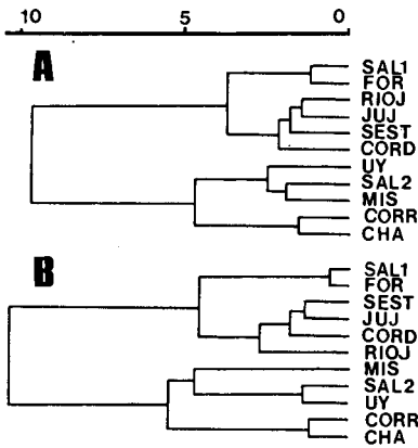
Fig. 3. Clasificaciones alternativas de OTUs de T. etheridgei y T. catalanensis , de distintas procedencias geográficas. Método WPGMA. A. Reducción proporcional con siete caracteres (CA5); B. Reducción proporcional mínima, con tres caracteres (CA6).
