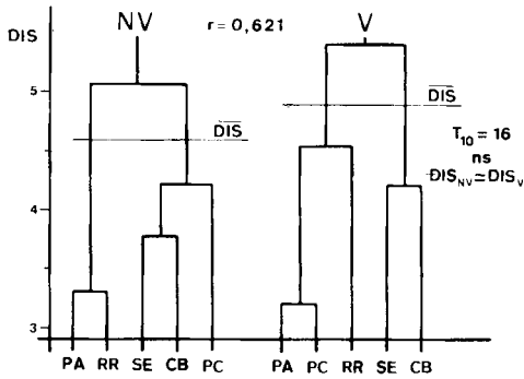
Fig. 7. Dendrogramas de afinidad global en el uso del espacio obtenidos a partir de distancias euclídeas inter-específicas: \overline{DIS} . Distancia euclídea media. Para abreviaciones ver figuras 3 y 6.
