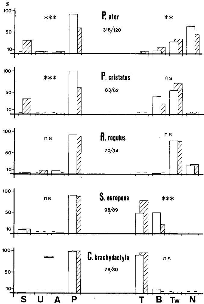
Fig. 1. Uso porcentual de Macrostratos y Sustratos del Pino con viento (▨) y sin viento (□) y resultados de los tests de la G. Bajo el nombre de las especies el número de muestras sin viento (izquierda) y con viento (derecha). S. Suelo; U. Arbustos; A. Aire; P. Pino. T. Tronco; B. Ramas > 1 cm de Ø; Tw. Ramas < 1 cm de Ø; N. Acículas; ***p < 0,001; **p < 0,01; ns. No significativa; - test no efectuado.
