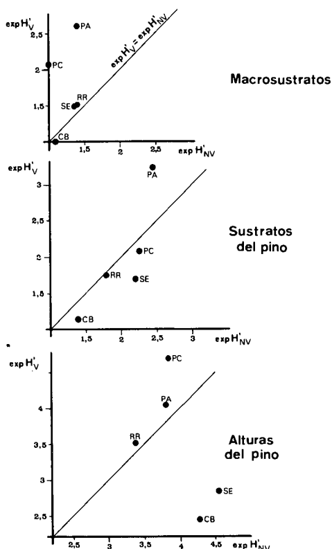
Fig. 5. Amplitud de nicho de las especies con viento ( \exp H'_v ) y sin viento ( \exp H'_{NV} ). Ver figura 3 para abreviaciones.
