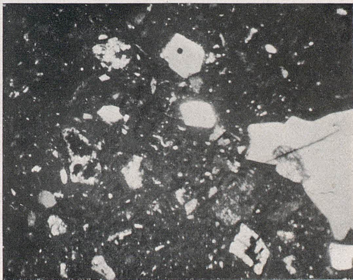
Fig. 2. — La misma entre nicoles cruzados
