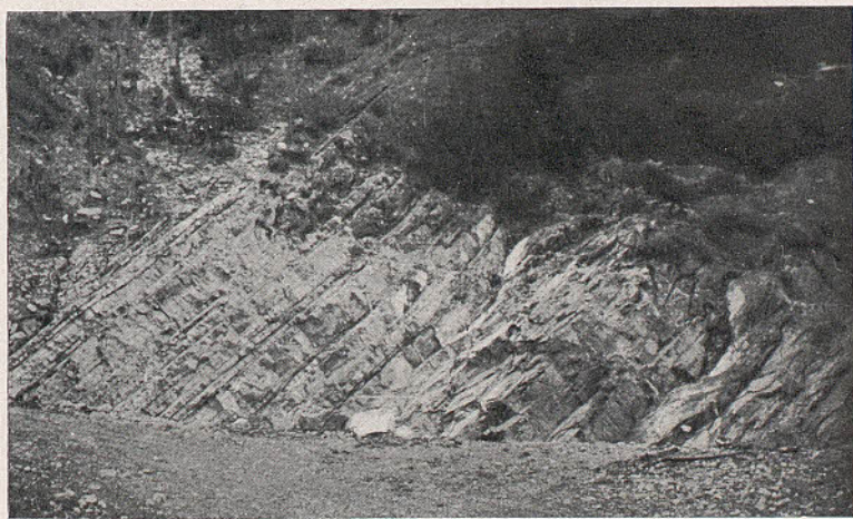
Fig. 2. — Riolita en lajas del borde de la colada ; camino de Greixa a la Font del Clot d'En Pere
