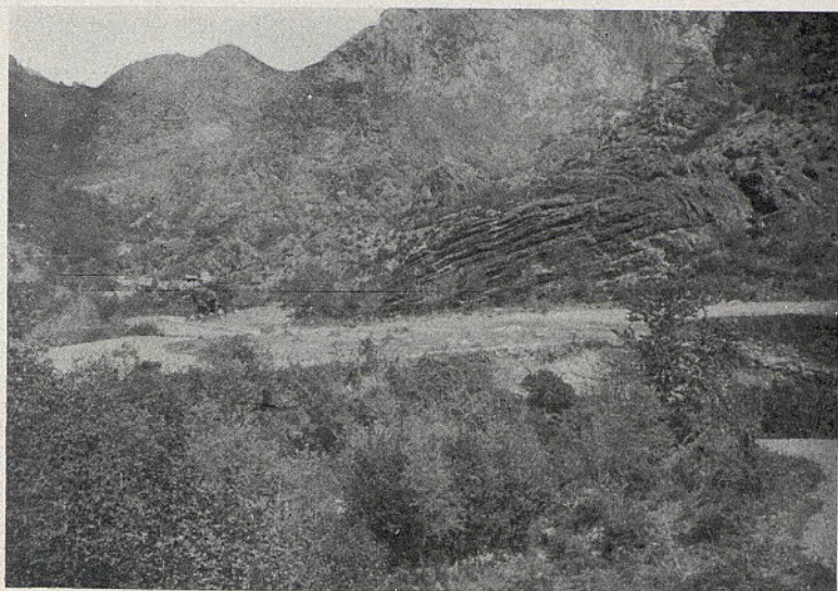
Fig. 1. — La colada al Este del Coll de Pilatos; en primer término, riolita en lajas del borde de la colada
