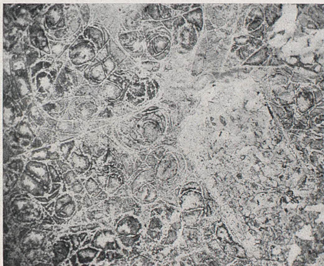
Fig. 2. — Riolita roja y verde, perlítica, de Greixa; L. ord. 15 d. Fenocristales de feldspato descompuesto, base perlítica
