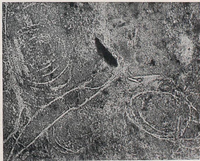
Fig. 2. — Riolita en lajas del borde de la colada, Greixa ; L. ord. 40 d. Perlitas conservadas en la pasta devitrificada a pesar de las grandes presiones que ha experimentado
