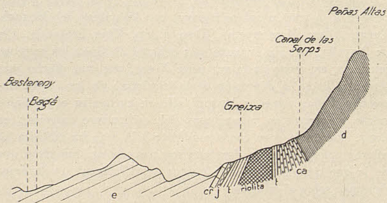
Fig. 3. — Corte geológico desde Bagá a Peñas Altas por Greixa. d. devónico; ca. carbonífero; t. permotrias; j. jurásico; cr. cretácico; e. eoceno
