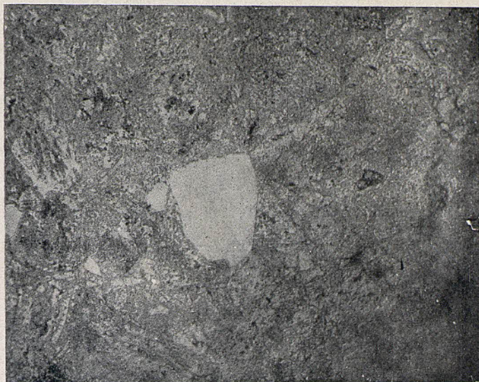
Fig. 1. — Brecha riolítica de Greixa ; L. ord. 15 d. Fragmentos de cuarzo y feldespato descompuesto ; ídem de riolita ; base de toba silicificada
