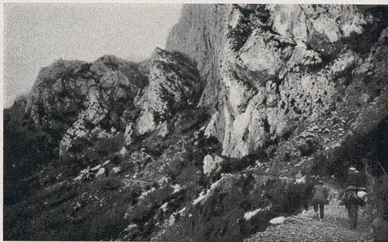
Fig. 2. — Camino de Greixa a la Font de la Cabrera. Calizas devónicas de la base de Moxaró
