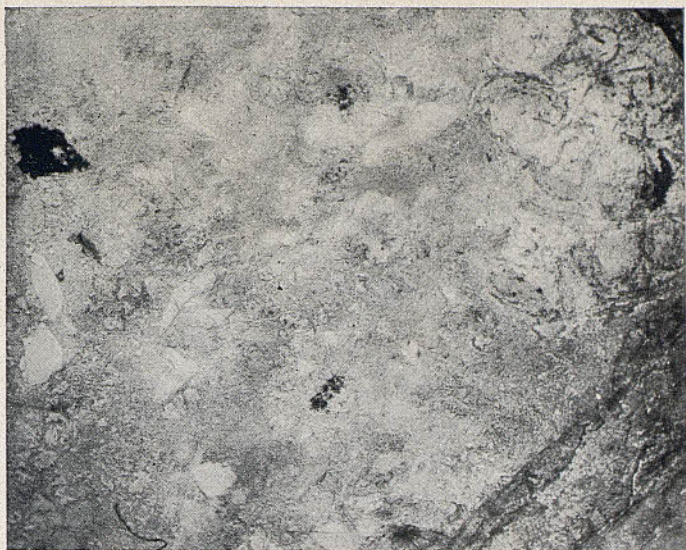
Fig. 1.—Toba riolítica del torrente del Forat. L. ord. 15 d. fragmentos angulosos de cuarzo, trozos de riolita perlítica; base felsítica silicificada
