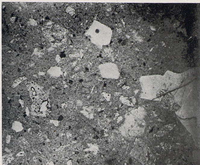
Fig. 1. — Riolita gris, Greixa; L, ord. 15 d. Fenocristales de Ortosa y cuarzo sobre base vítrea en la que destacan granillos de cuarzo y laminillas de mica
