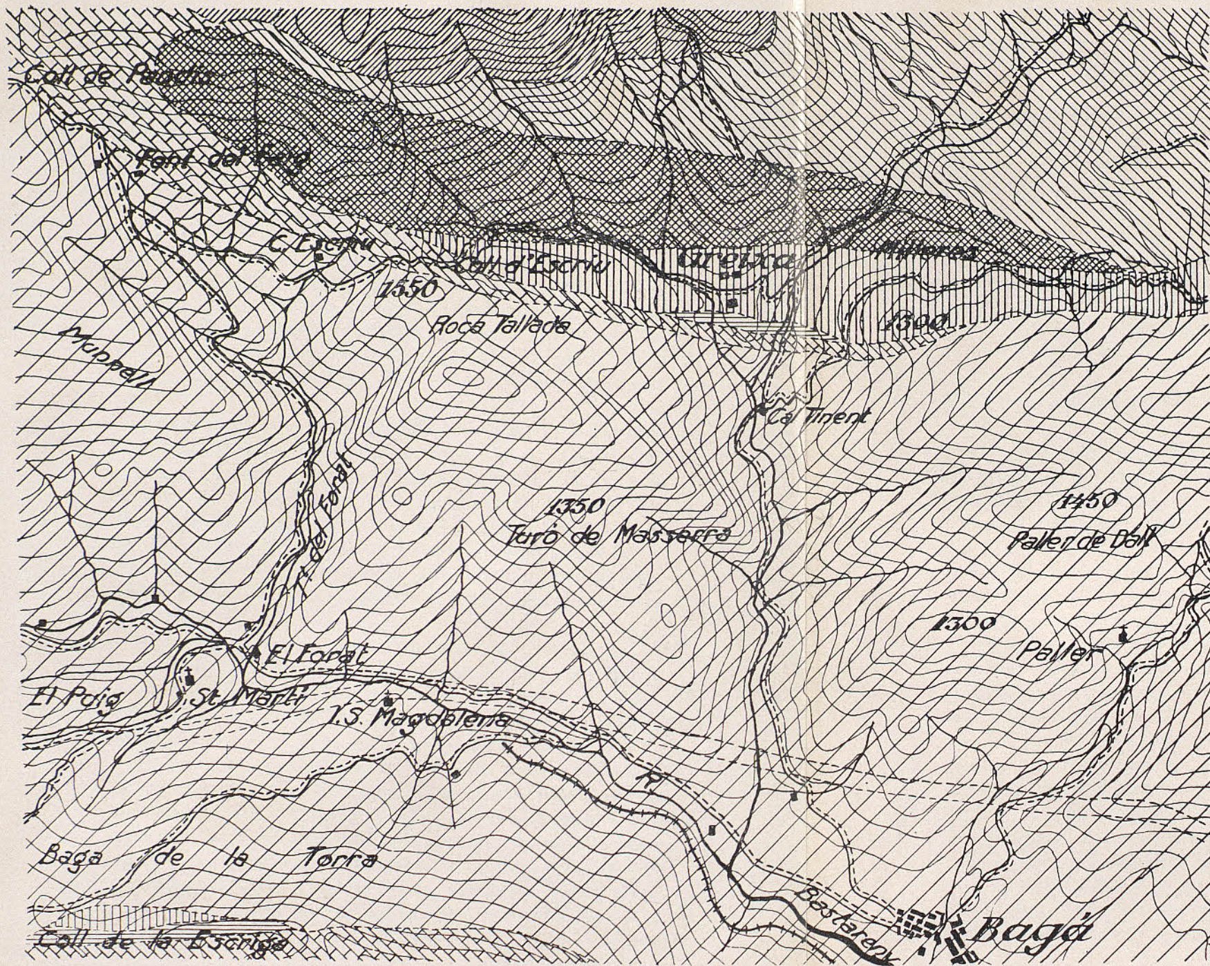
Fig. 1. Mapa geológico de los alrededores de Greixa
