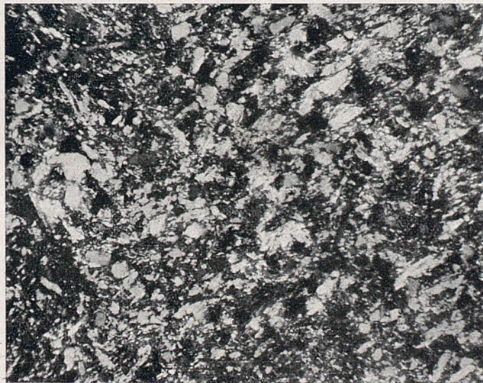
Fig. 2.—Igual roca; nicoles cruzados 15 d. Algo de mica y base felsítica
