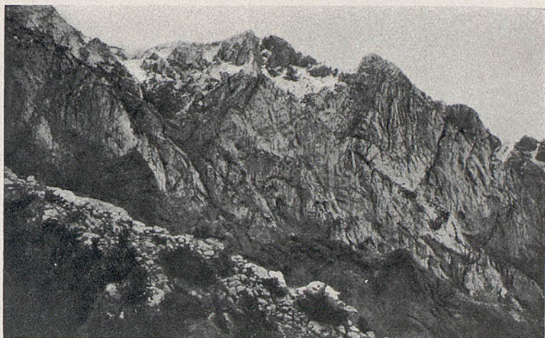
Fig. 1. — Masa de riolita entre el barranco que nace en el Coll del Escriu y el pie del Moxaró
