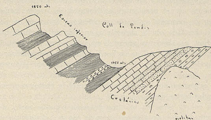
Fig. 9. — Terminación de la erupción cerca del Coll de Pendís y terrenos con ella relacionados
